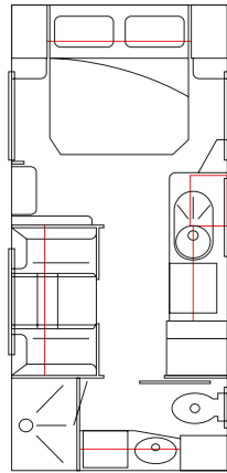
19'6" MID DOOR
