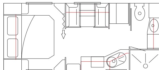
20' MID DOOR
